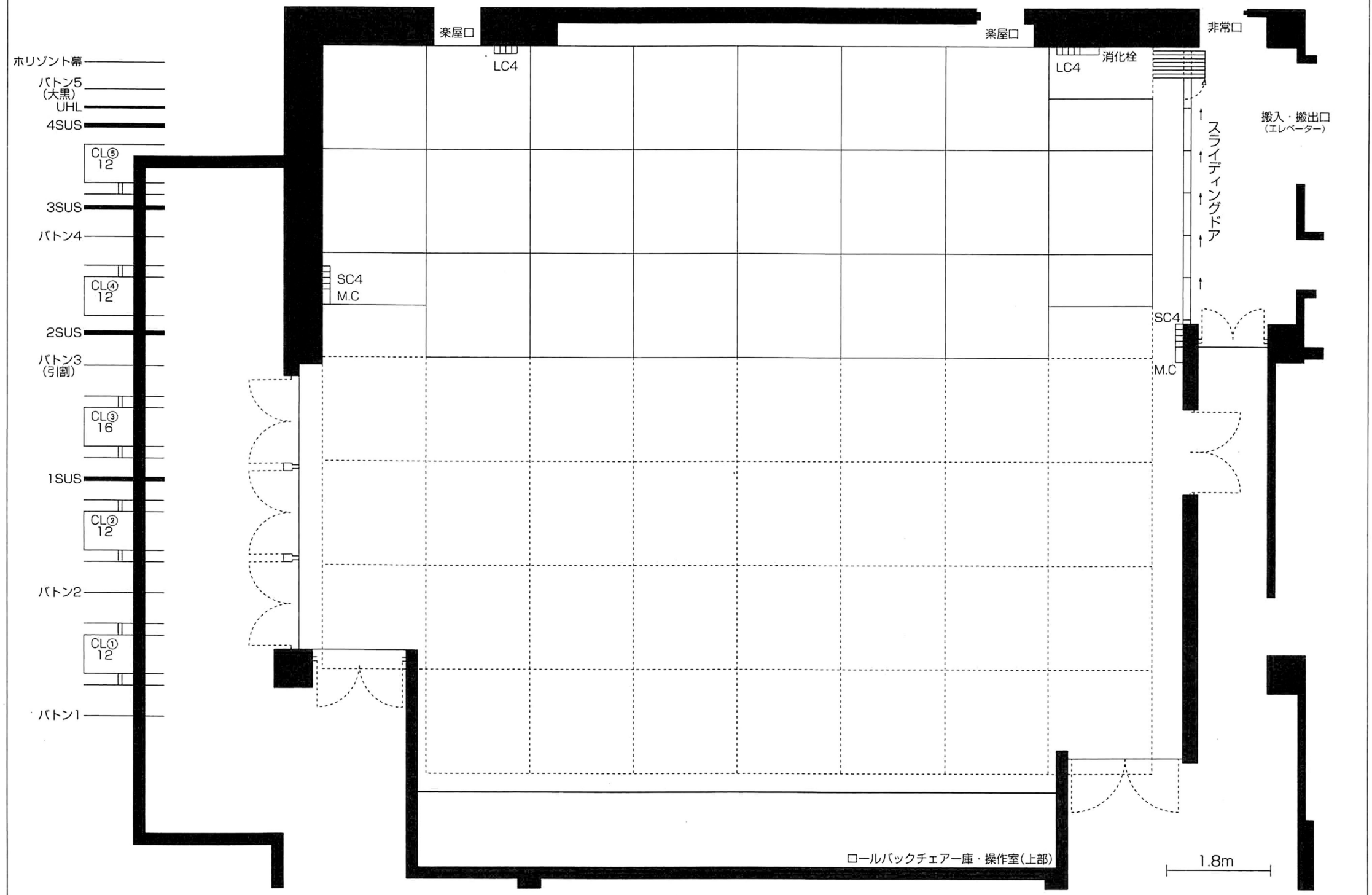
プラネットホール舞台平面図
